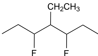
4-ethyl-3,5-difluoroheptane
