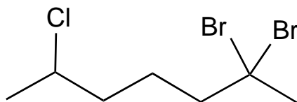
2,2-dibromo-6-chloroheptane
