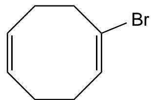
1-bromo-1,5-cyclooctadiene
