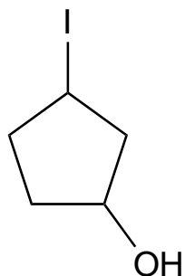
3-iodocyclopentanol
